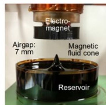
磁性流体液錐の頂点位置決め制御
